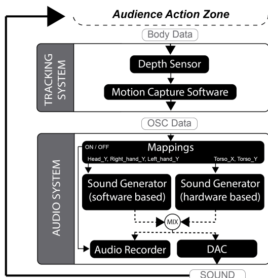
Figura 6: Arquitetura do sistema Présence
