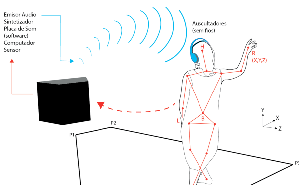
Figura 3. Esquema geral do fluxo de informação do sistema.
