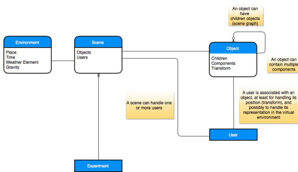
Figura 2 - Sistema relacional de Cena.
