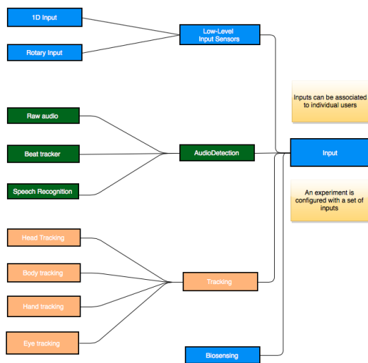
Figura 4 - Sistema de entradas através de dispositivos HID.
