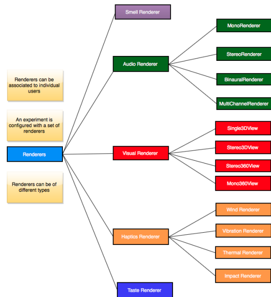
Figura 5 - Diferentes tipos de renderers.
